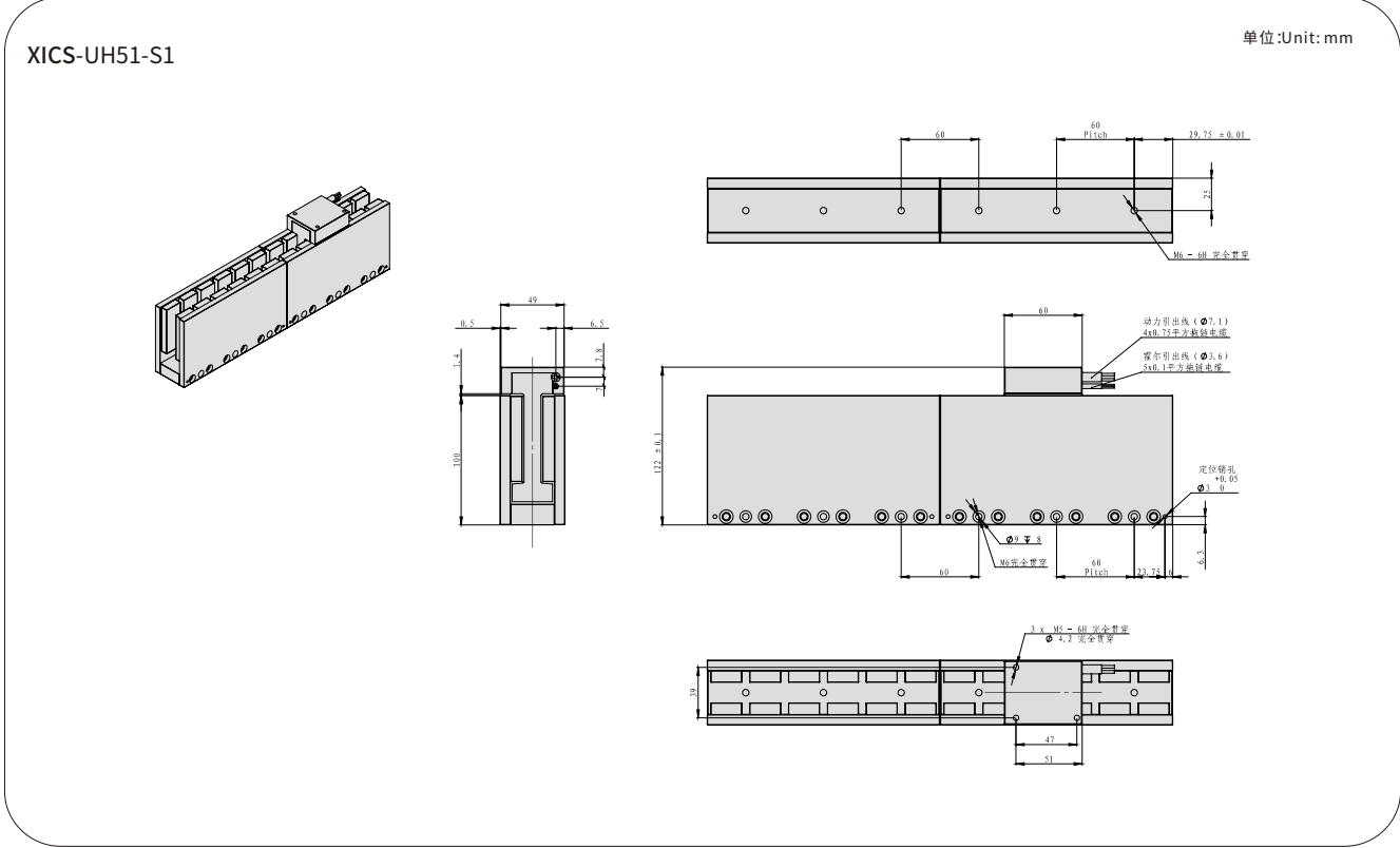
XICS 动 定子尺寸图 XICS Dimension diagram of Mover & stator
